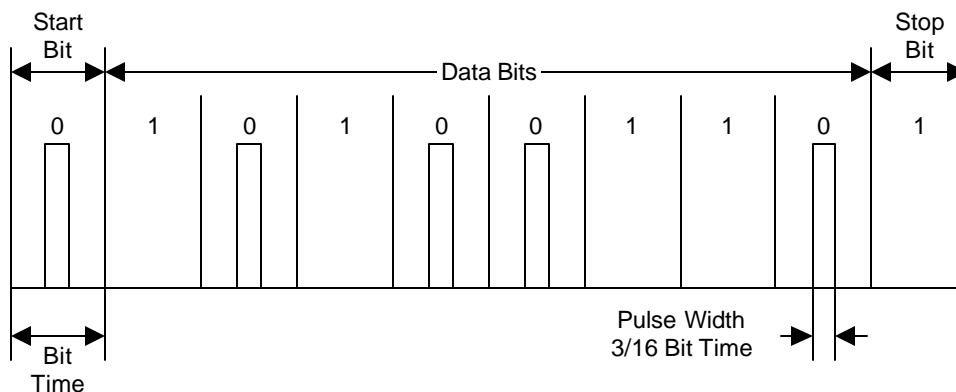
Figure 2. IR Byte
