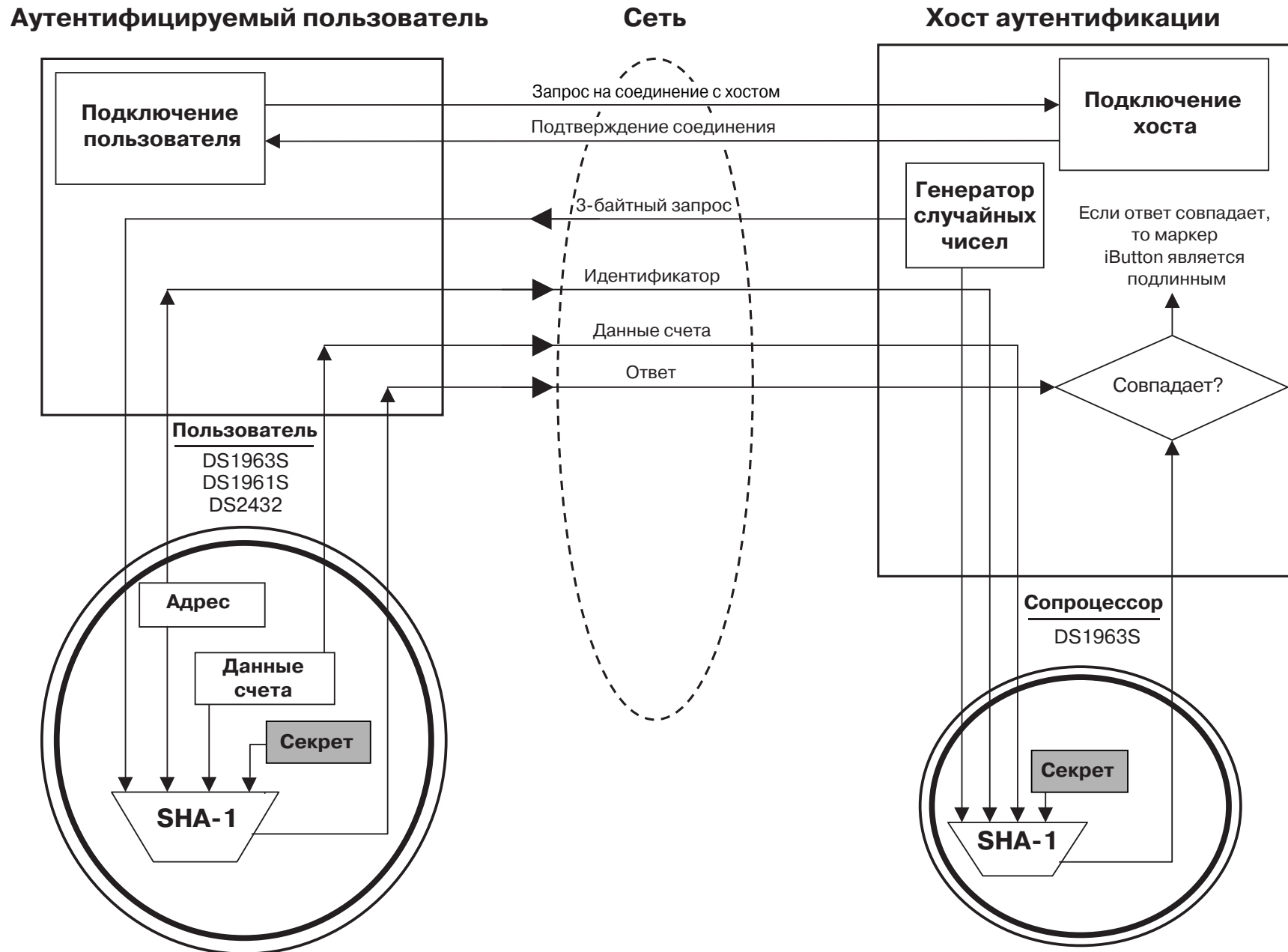
Рис. 3. Пример аутентификации «RemoteAuth»
