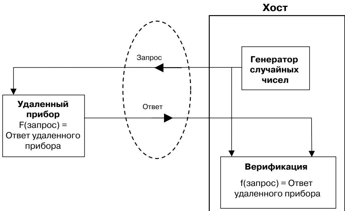
Рис. 1. Запрос—ответ
