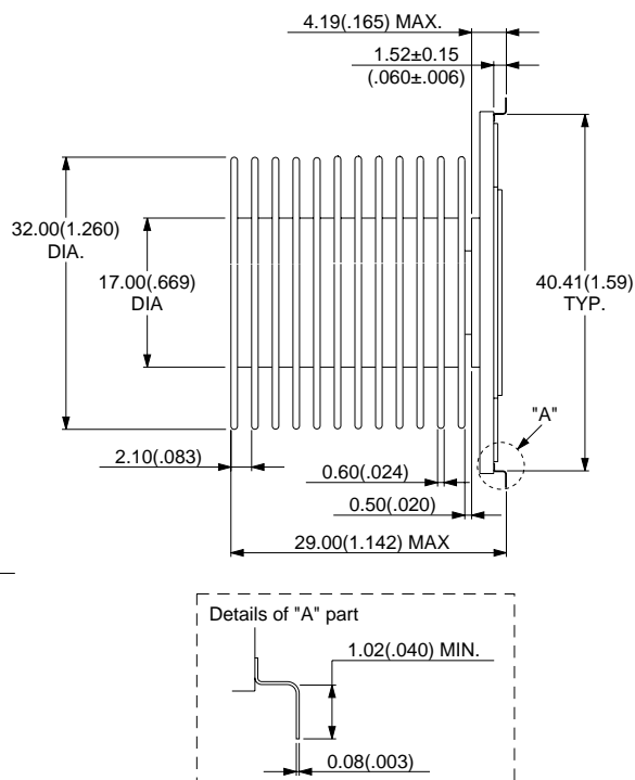
0.76(.030) 0.51(.020) 0.71(.028) 0.20(.008) INDEX AREA 37.08(1.46) 4.06(.160) 3.56(.140) 41.15±0.51(1.62±.020) 43.69±0.51(1.72±.020) 0.75(.030) MIN.
