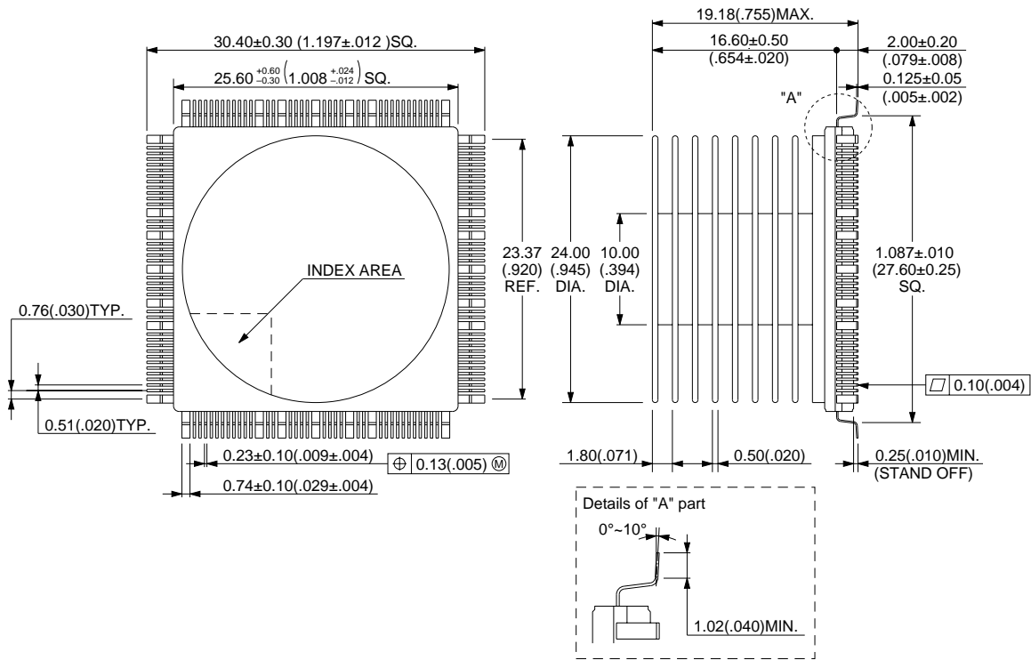
164-pin ceramic QFP (FPT-164C-C01)
