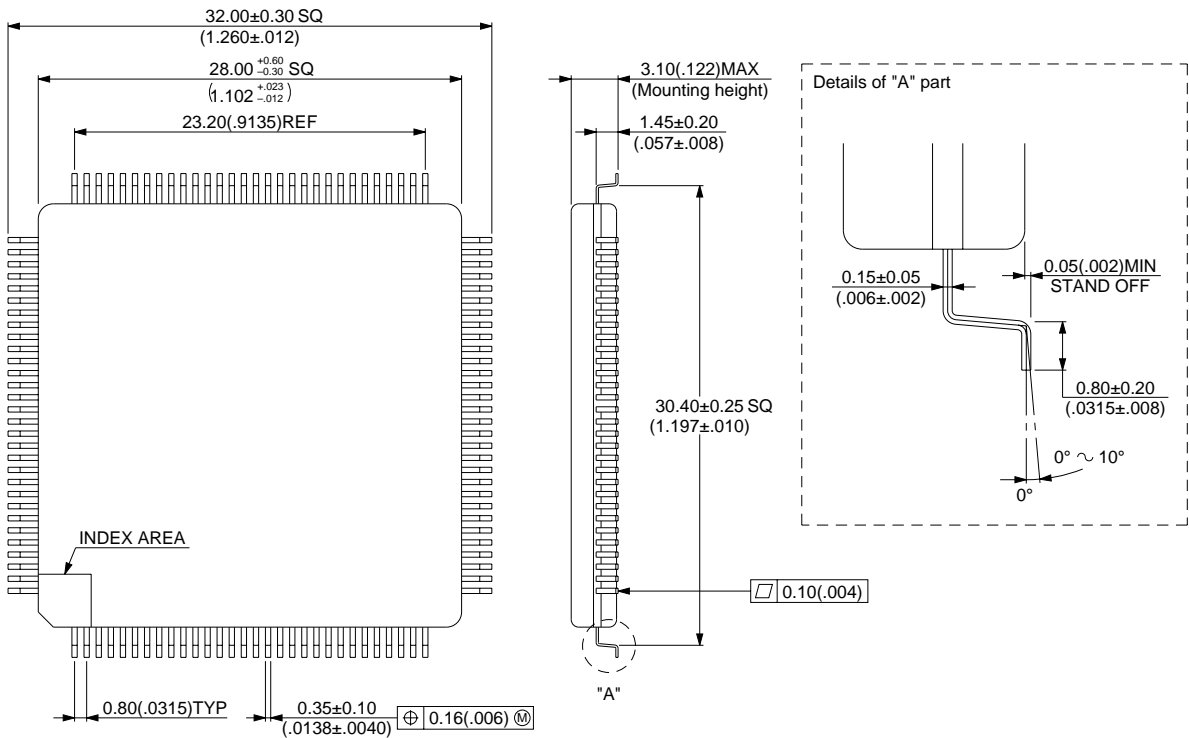
120-pin ceramic QFP (FPT-120C-C01)
